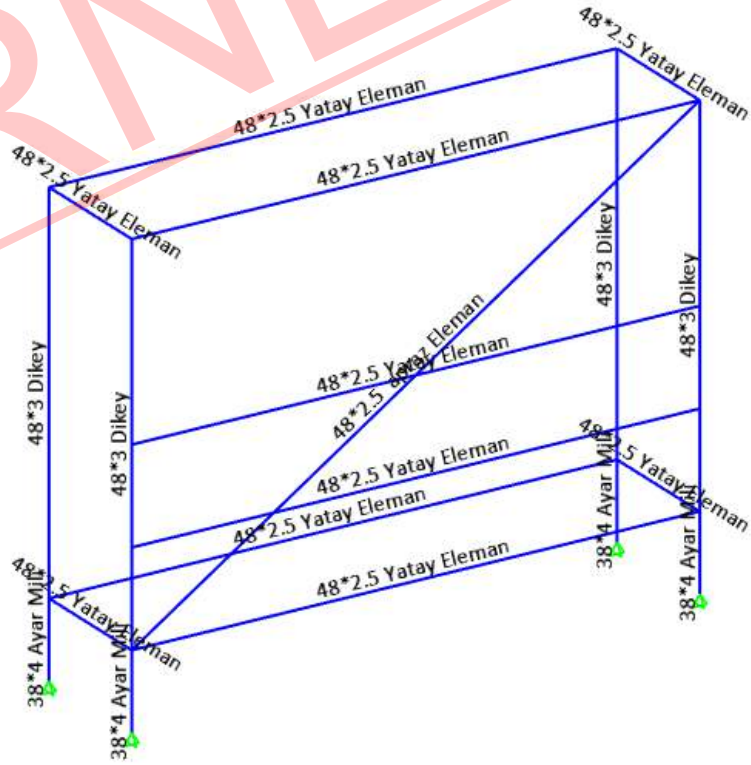
Şekil 1.5. Elemanların Kurulum Düzenleri
